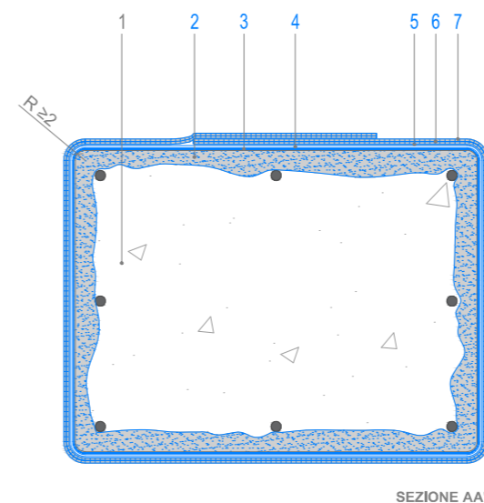
SEZIONE AA'
