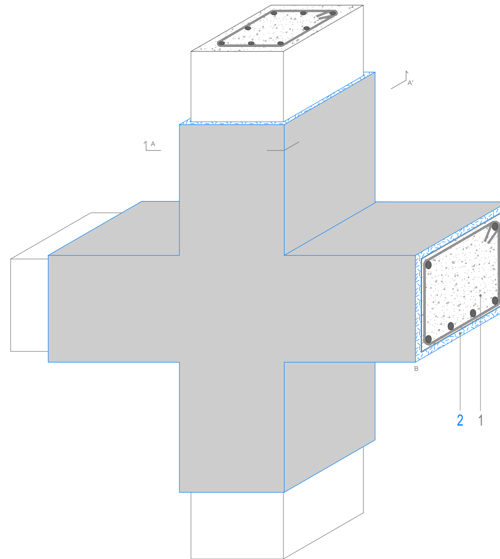
VISTA ASSONOMETRICA
