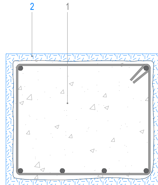
SEZIONA BB'
