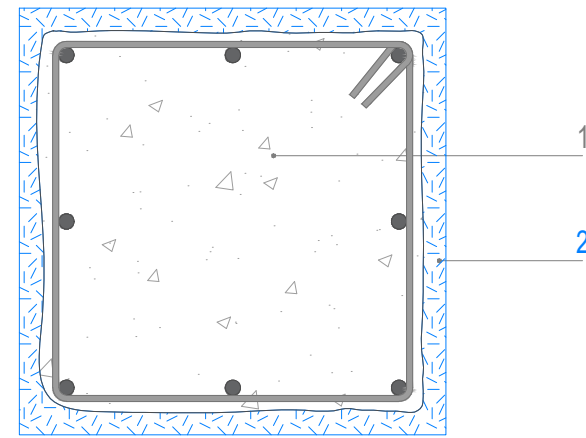
SEZIONA AA'
