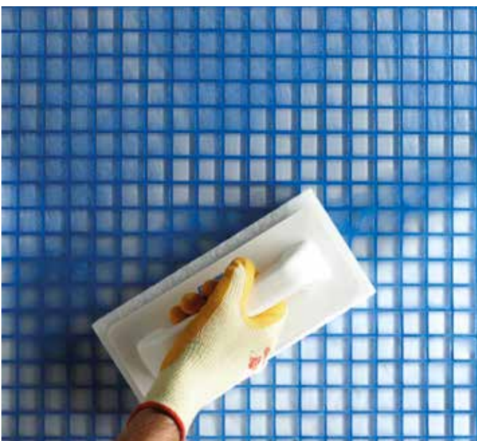
Pulizia del mosaico vetroso dopo la stuccatura
