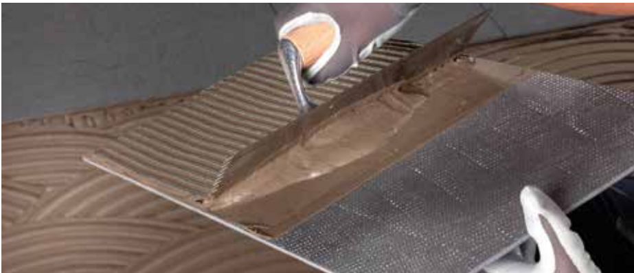
Posa di piastrelle sottili con tecnica della doppia spalmatura
