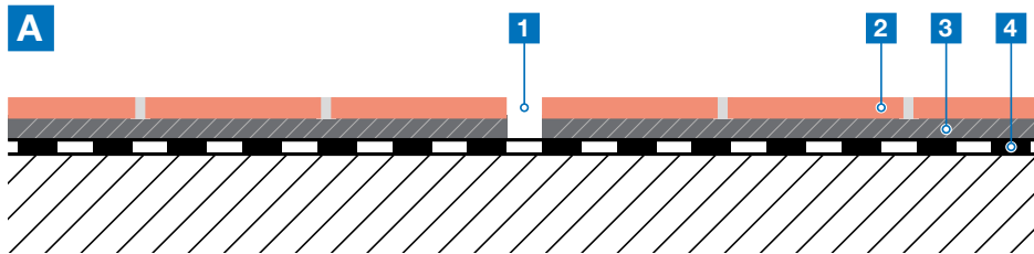
Rivestimento nuovo con giunto di dilatazione
