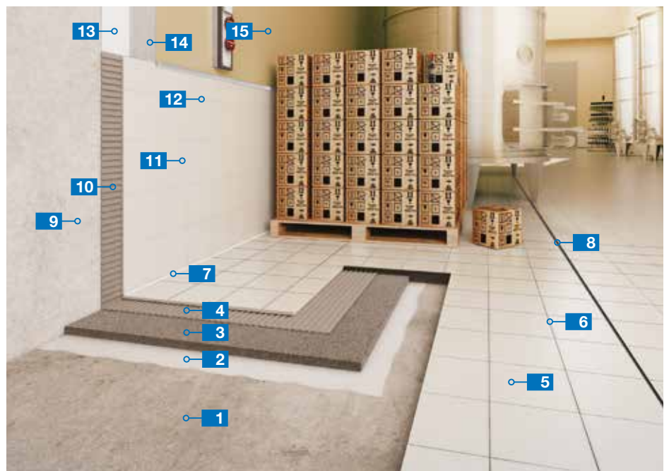
Sistema per la posa di ceramica in ambienti soggetti a traffico intenso ed aggressioni chimiche
