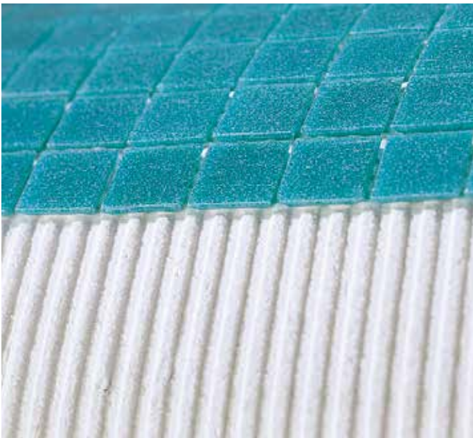
Posa di mosaico con adesivo ADESILEX P10
