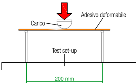
1. Test set-up per determinare la flessibilità di adesivi con strato sottile sulla base della deformazione
