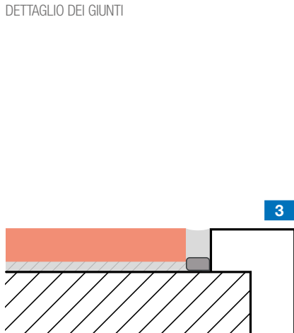
Giunti all'interfaccia con altri elementi
