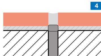
Giunto strutturale, solitamente sigillato con specifici profili e/o coprigiunti
