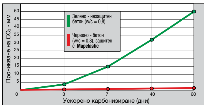
Фиг. 2: Защита с Mapelastic срещу ускорено карбонизиране (30% CO 2 ) върху порьозен бетон
