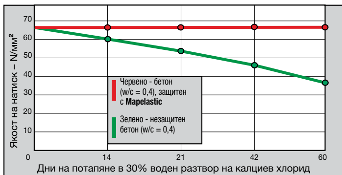
Фиг. 4: Защита с Mapelastic срещу намаляване на механичната якост на бетона, в следствие на калциев хлорид, който е съставна част на противозамръзващи соли
