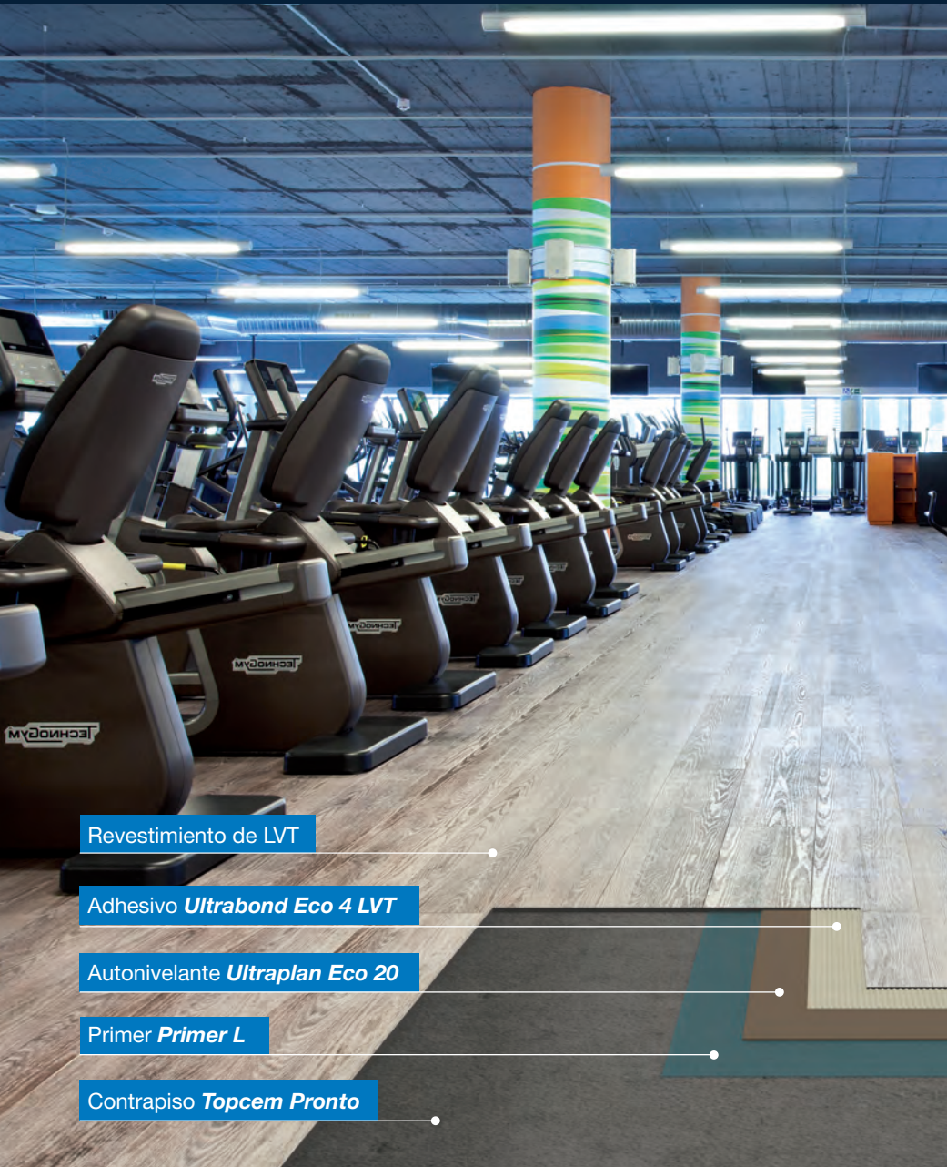
Sistema autonivelante para dar planicidad
