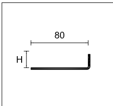
CPLB/2 Gestanzter Schenkel für die Verlegung in Fliesenkleber
