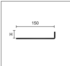
CPLB Trägerprofil für Aufsteckblende
