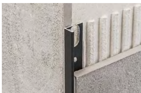
ZA/10 Aluminium Schwarz eloxiert
