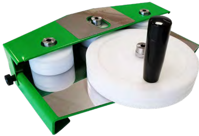
PROFLEX MASCHINE - Biegemaschine zum Biegen der Proflex Profile
