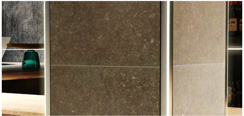
ZQAL/10B Aluminium Natur + ZQAL/10 PVC (opalineartig) Weiß glänzend
