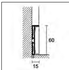
87/6 + 88/16SF Einsatz in Aluminium
