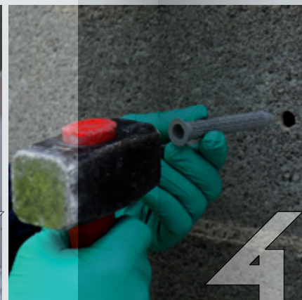
4 Вставьте в отверстие сетчатую втулку с подходящим диаметром и длиной
