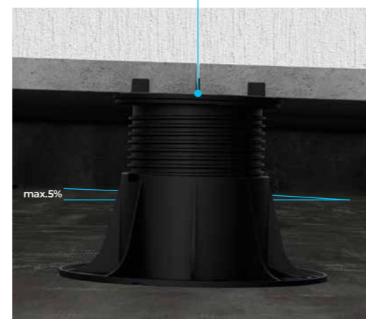
FIXNÁ HLAVA
