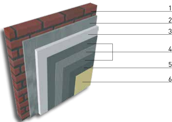
Schéma kontaktného zatepľovacieho systému MAPETHERM
