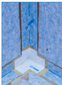
Détails de l'imperméabilisation d'un angle intérieur avec Mapeguard IC
