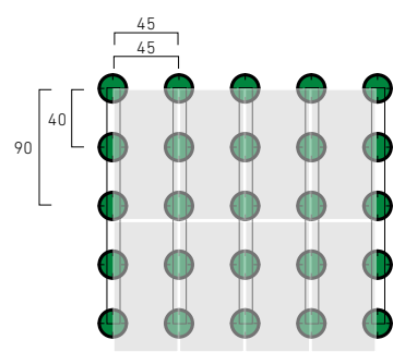
45 x 90 Trafic piétonnier élevé Hoher Fussgängerverkehr
