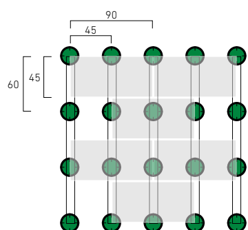
45 x 90 Trafic piétonnier léger Niedriger Fussgängerverkehr
