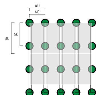
40 x 80 Trafic piétonnier léger Niedriger Fussgängerverkehr
