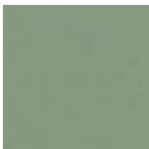
Grønn nr. 73
